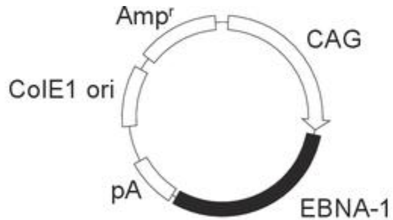
pCXB-EBNA1 6.4 kb
