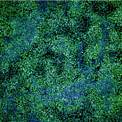
SOX17 + DAPI
