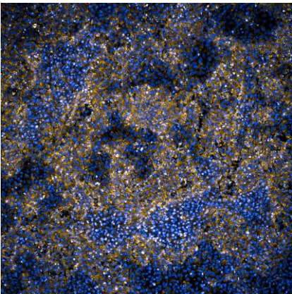
CXCR4 + DAPI
