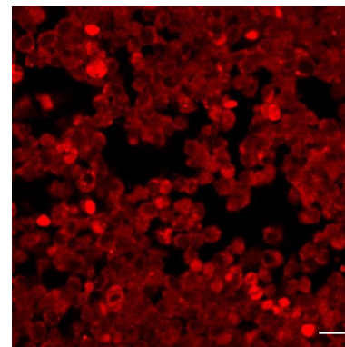
Brachyury
