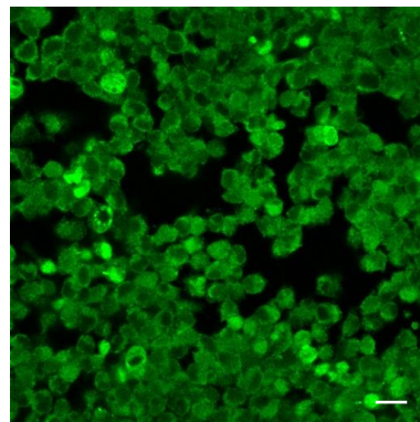
Nkx-2.5
