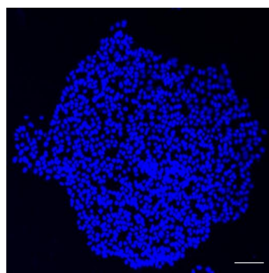
DAPI
