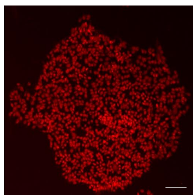
TRA-1-81
