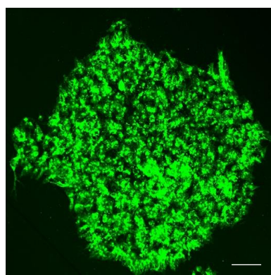
SSEA4
