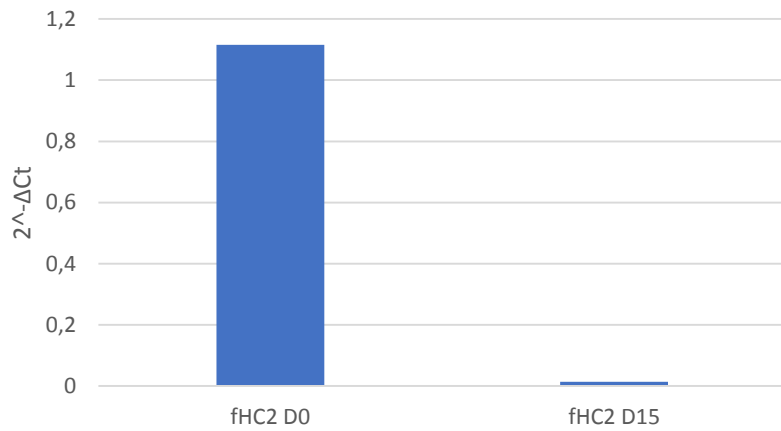
OCT4
