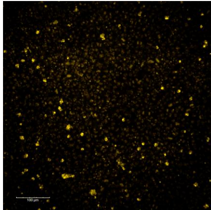
CXCR4
