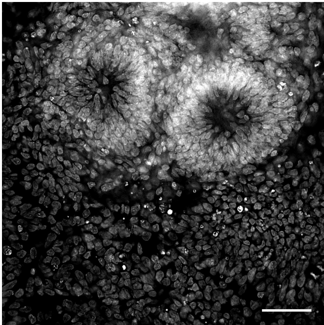
Hoechst
