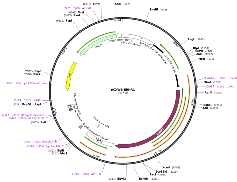
pCXWB-EBNA1
